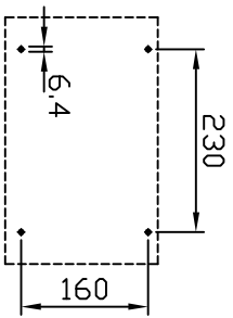
Bohrbild
